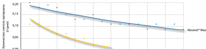
Сравнение производительности Abranet® Max и стандартной ленты на бумажной основе в градации зерна P120 – Шлифование дуба
